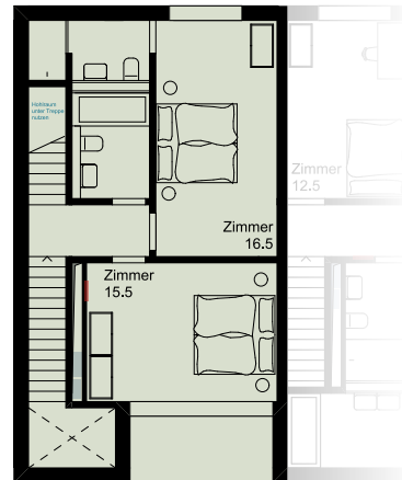
1. Obergeschoss
